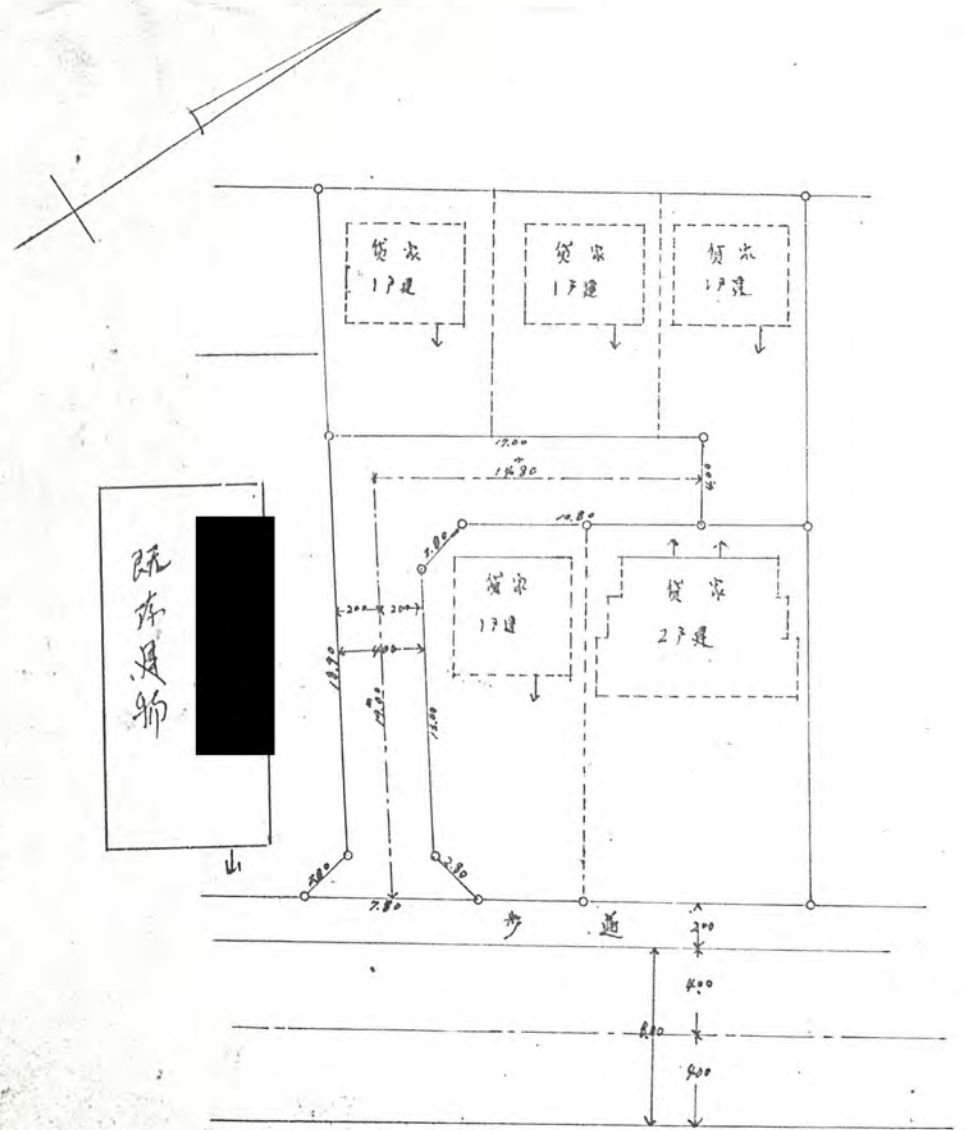
測量図 5/300
