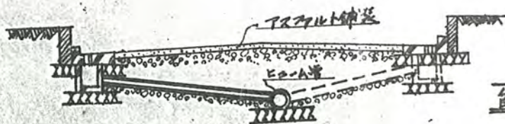
A~A'構造図 1/500
