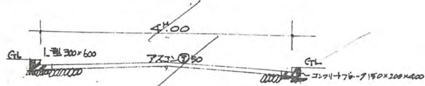
道路断面図 1/50
