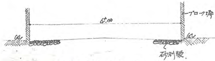
道路断面図 1/50
