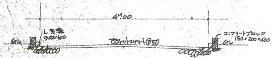
道路断面図 1/50
