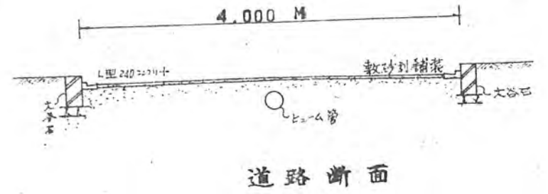
道路断面
