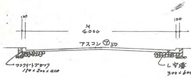
道路断面図 1/50
