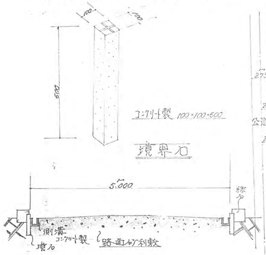
道路断面図 1:50
