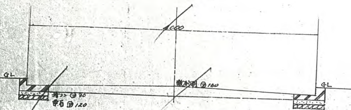
断面図
