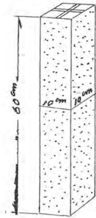
標杭ノ図
