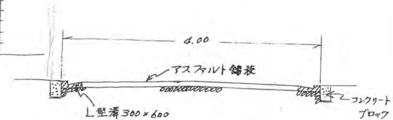
道路断面図
