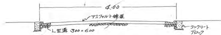
道路断面図
