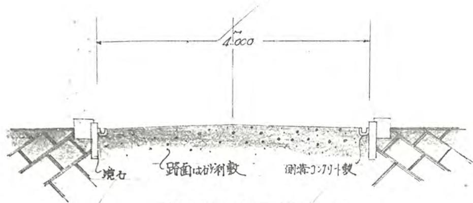
道路断面図 1:50
