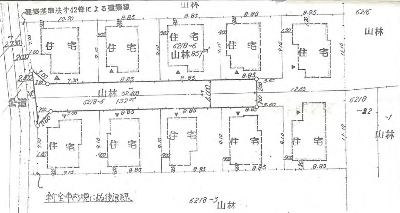
配置図 S=1/300
