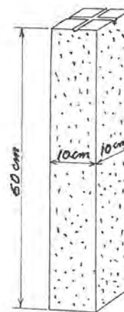
標杭ノ図
