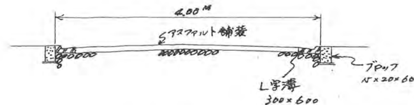
道路断面図
