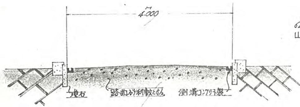
道路断面図 1:50
