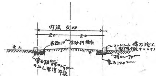
道路断面図 5:100
