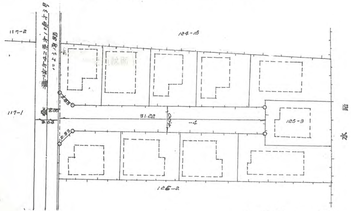
地籍図 S=1:300
