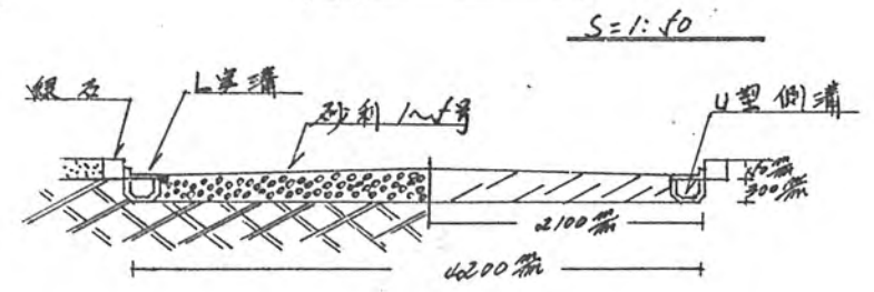
道路断面図
