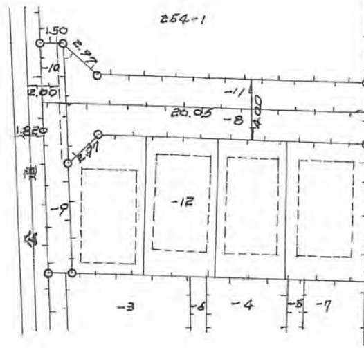
地籍図 S=1:300
