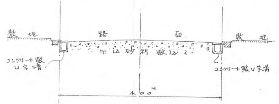
構造図 1/50
