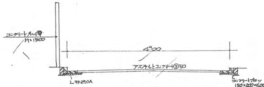
道路断面図 1/50
