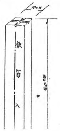
境界石断面図
