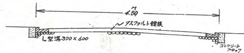
道路断面図 s=1:50
