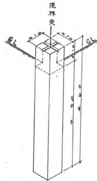
界標石図 S=1:10
