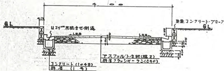
構造図 S=1:50
