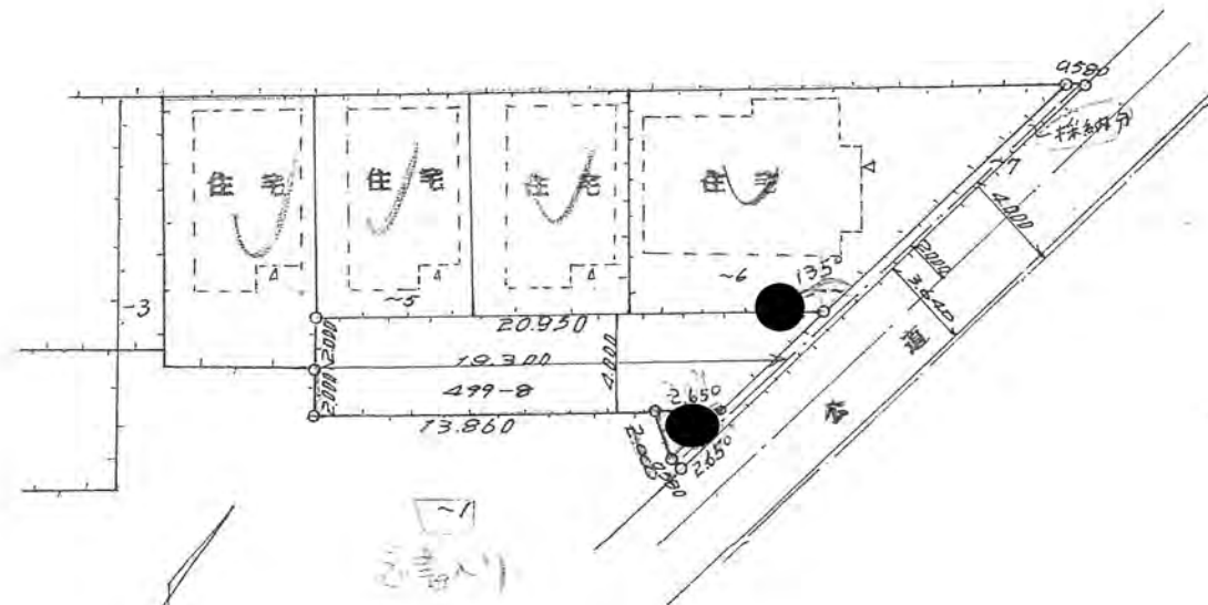
地籍図 S=1:300
