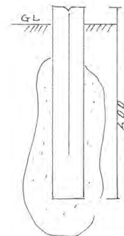
境石断面図 1:10
