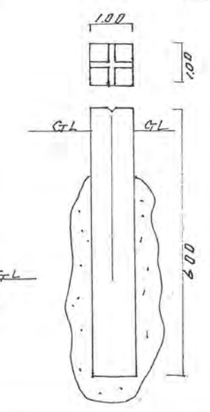
境石構造図 1/50
