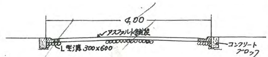
道路断面図
