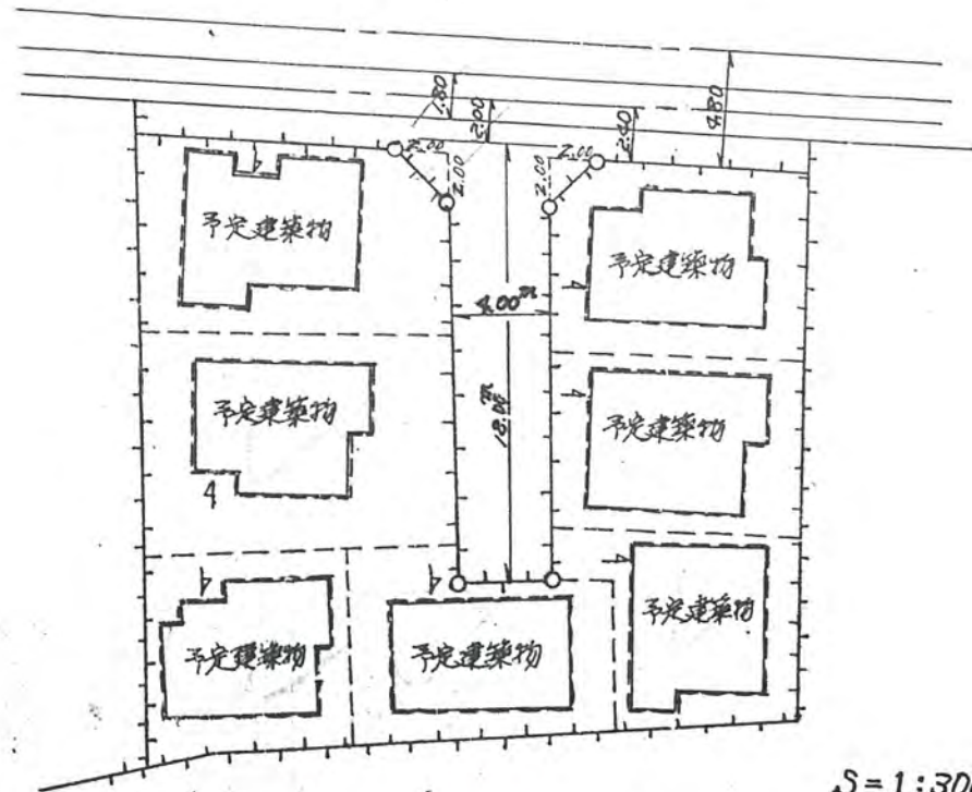
構造図
