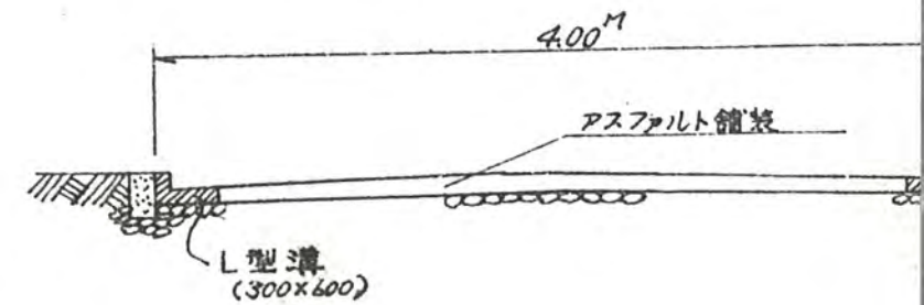
道路断面図 S 1:50
