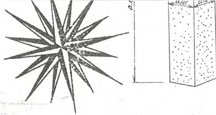
標杭ノ図 S 1:10
