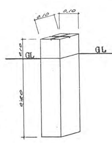
道路位置標識 SCALE=1/10
