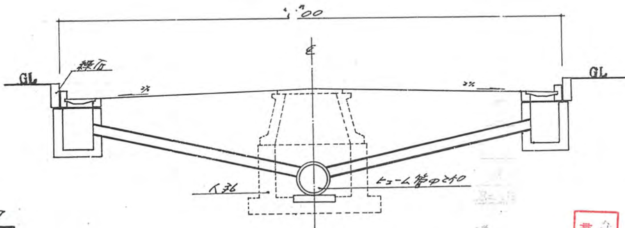
道路構造圖
