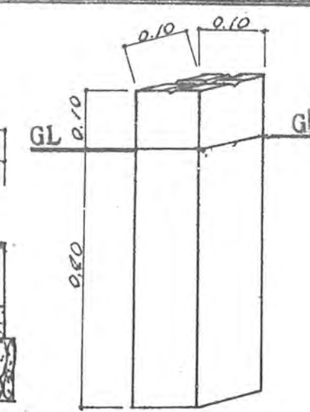
標識図 SCALE=1/10
