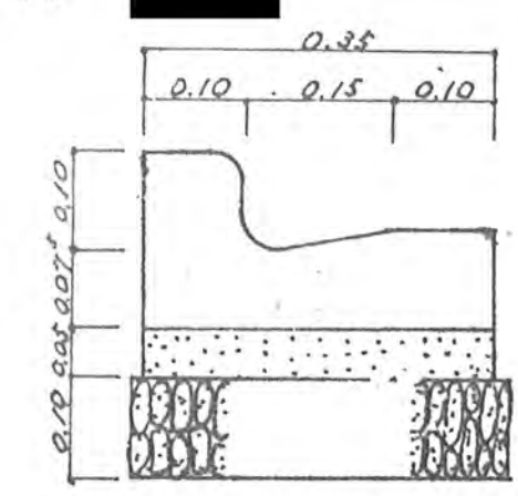
L字溝構造図 SCALE=1/10
