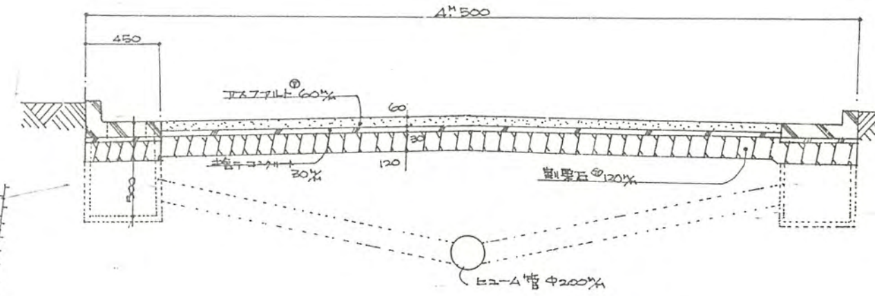
構造図
