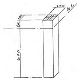
標示杭 S. 1/20
