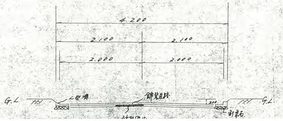
横断図
