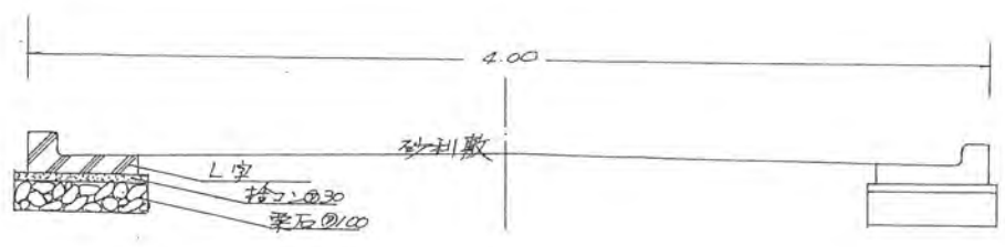
断面図 S=1:30
