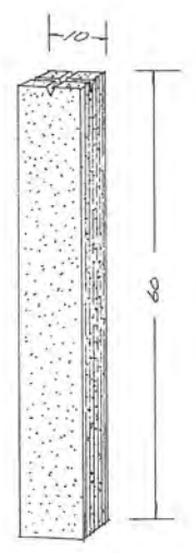
構造図 S=1:10
