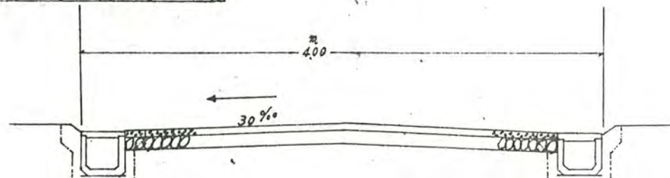
A~B 道路構造図 1/40
