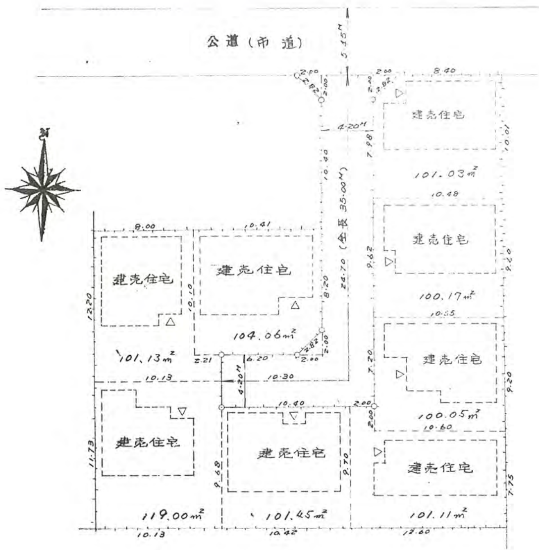
地籍図 S = \frac{1}{300}
