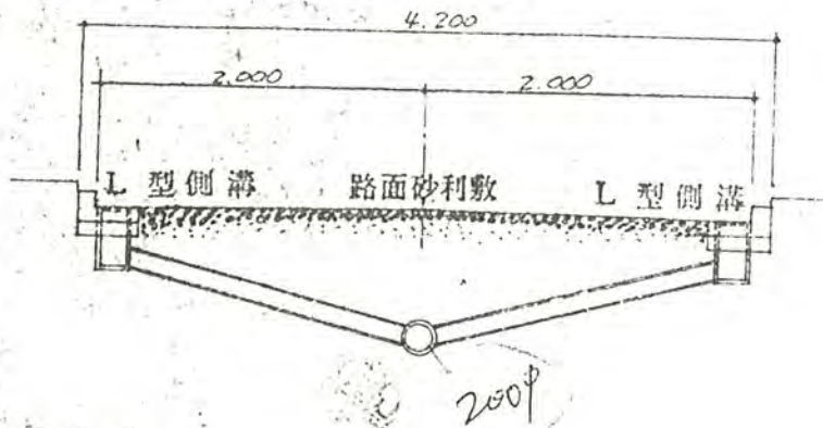
道路断面図 S = \frac{1}{50}
