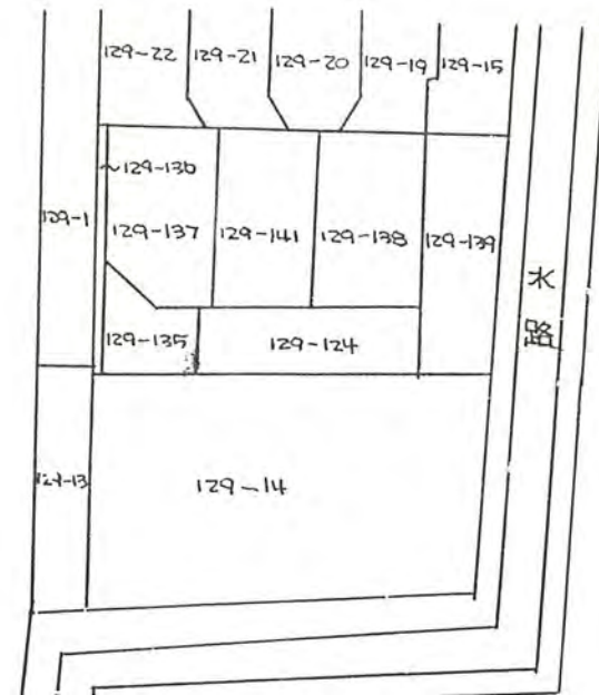
地籍図 1/300
