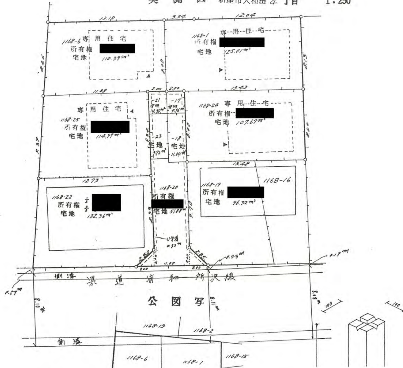
実測図 新座市大和田4丁目 1:250
