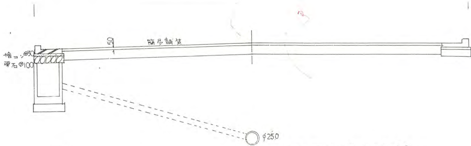
道路断面图 S = 1:30
