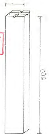
境石構造図 S=1/10
