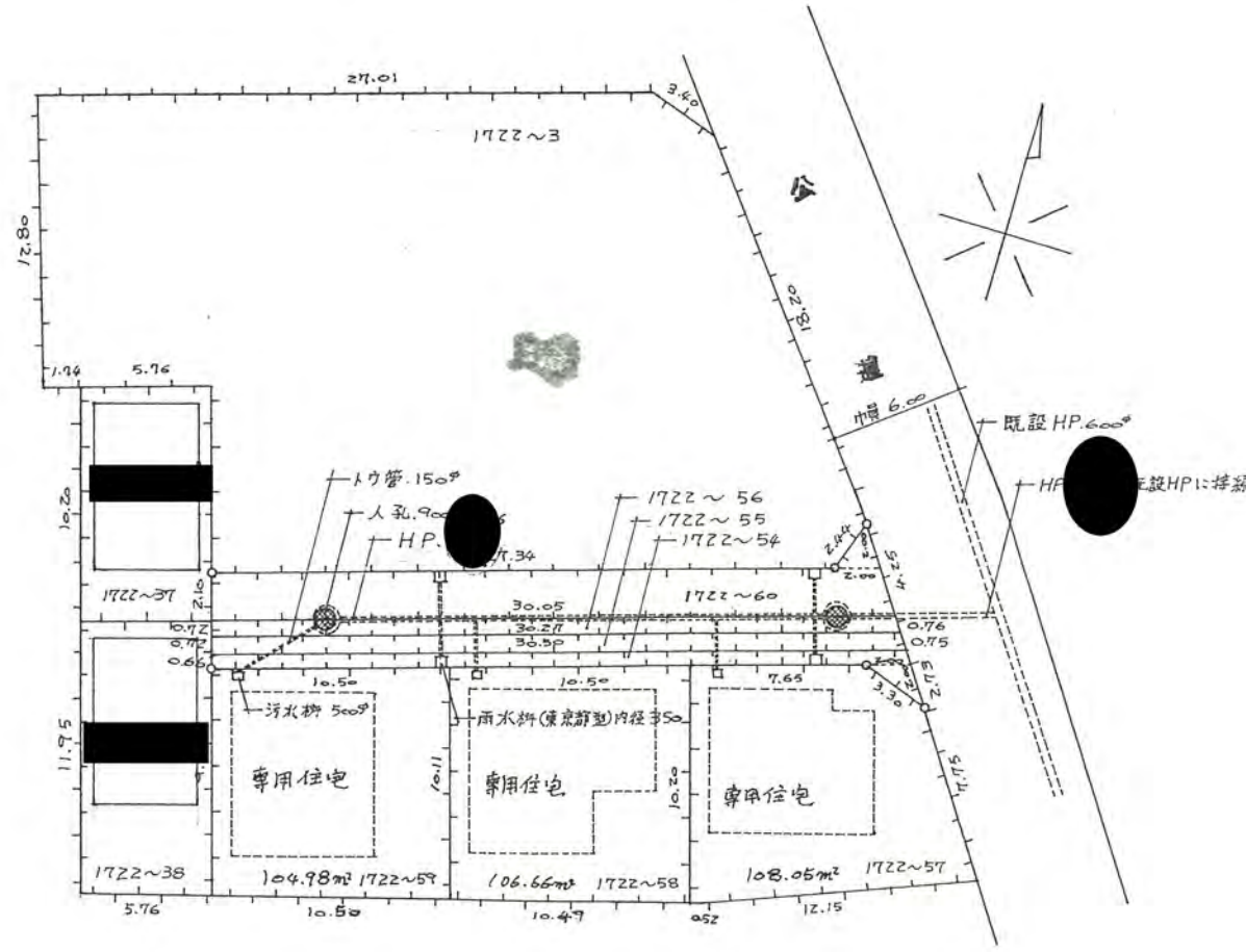
地籍図 S1:300
