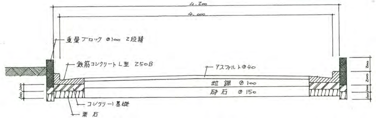
構造図 S1:30
