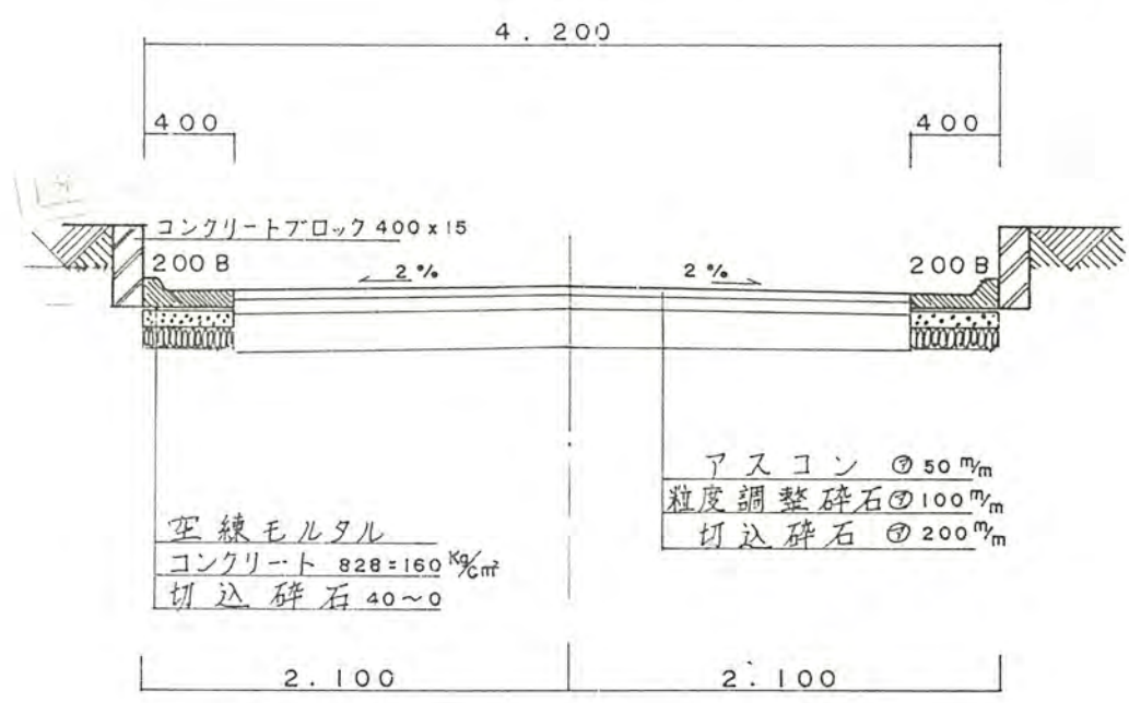
構 造 図
