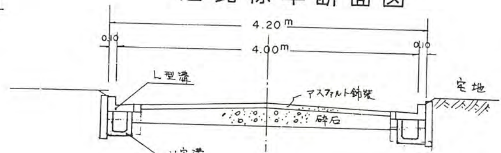
道路標準断面図
