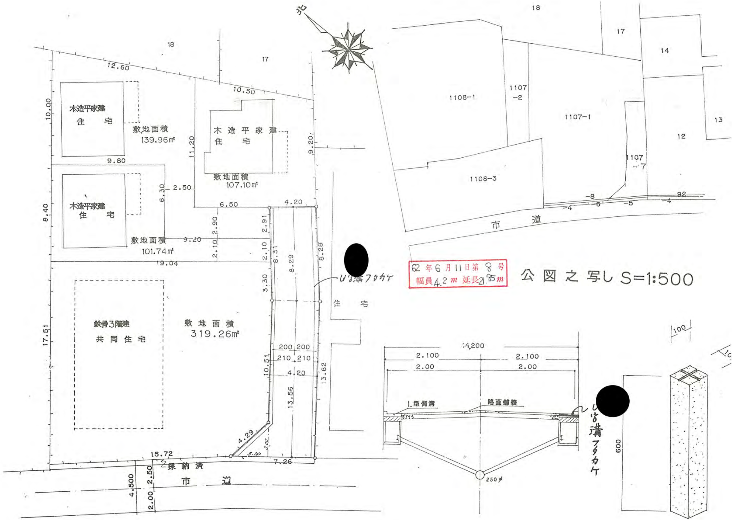
構造図 S=1:200
