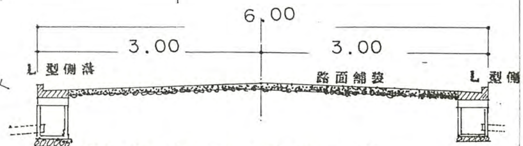
道路断面図 S=1/30
