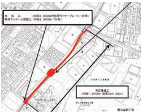
工事概要図
