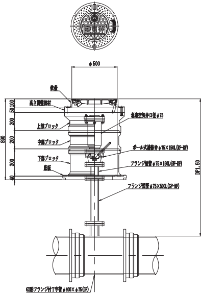
レジンコンクリート製 急速空気弁室
