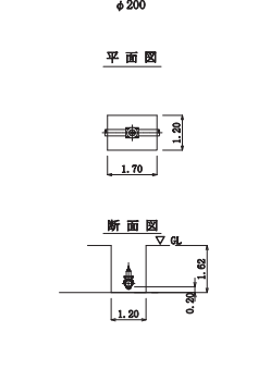
不断水弁設置工土工図
