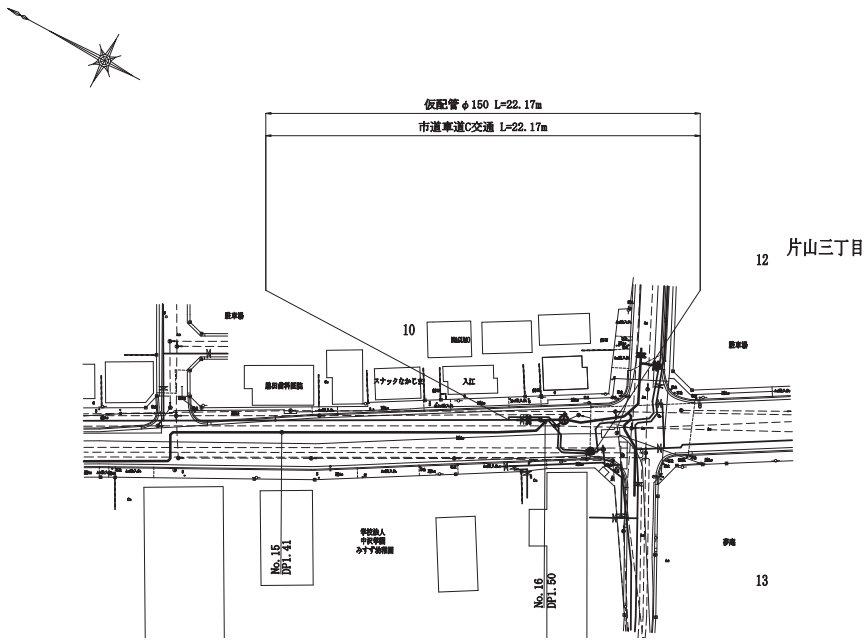
仮設平面図 S=1:500
