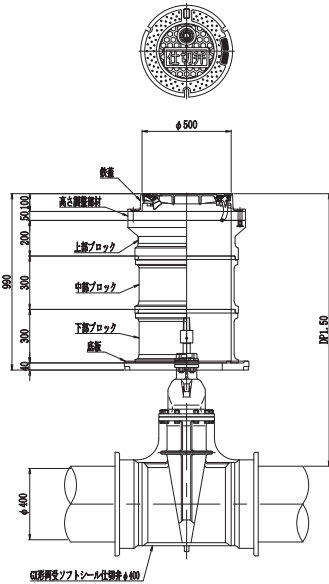
レジンコンクリート製 φ 400仕切弁室
