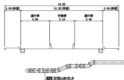
横断面 S=1:100
