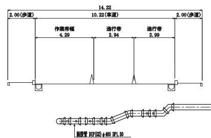
横断面 S=1:100
