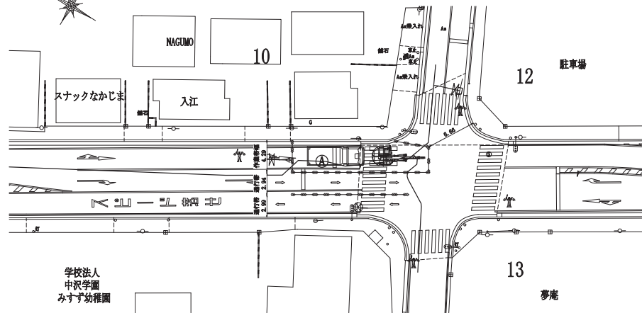
交通規制図②（参考図） S=1:250
