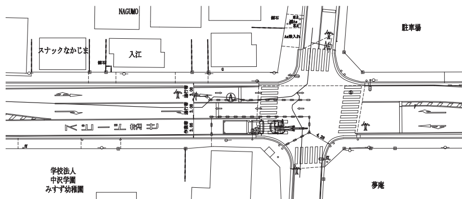
交通規制図③（参考図） S=1:250
