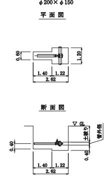
不断水分歧工土工図
