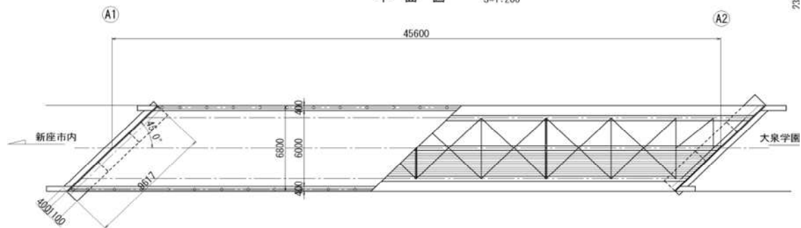
平 面 図 S=1:200
