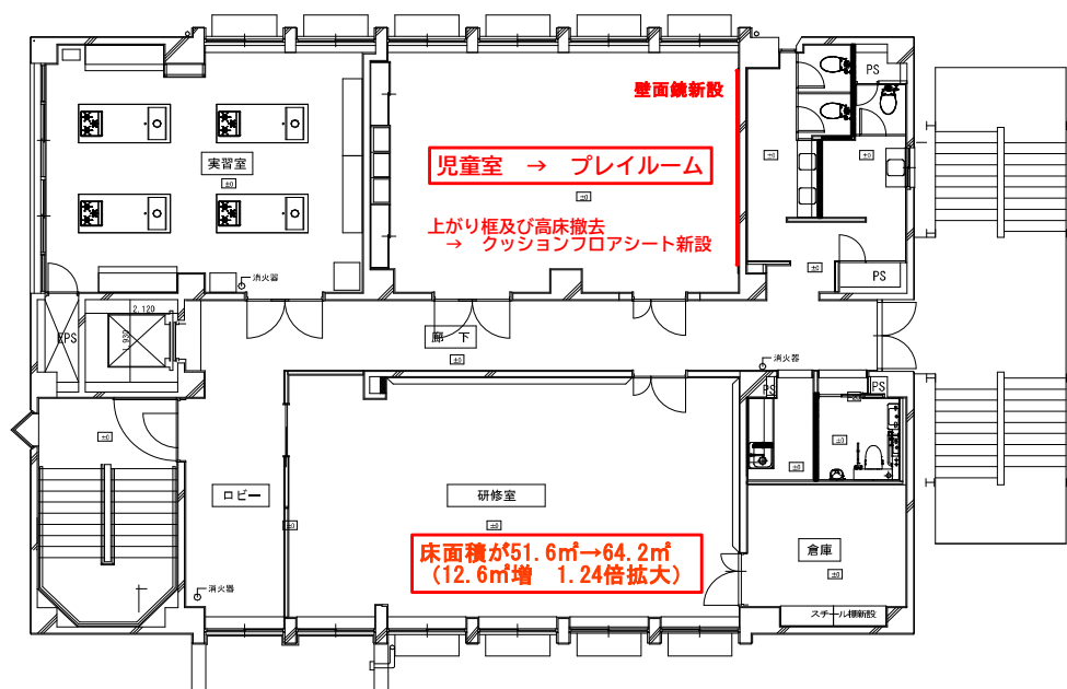
2 階平面図
