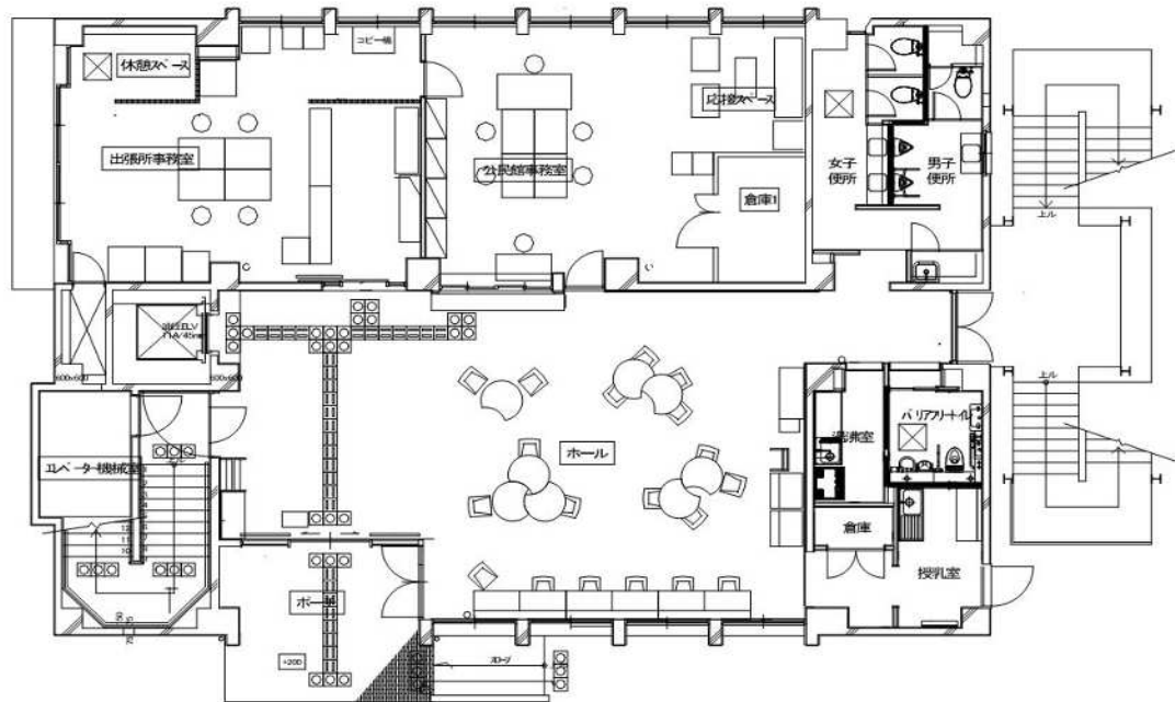
1 階平面図
